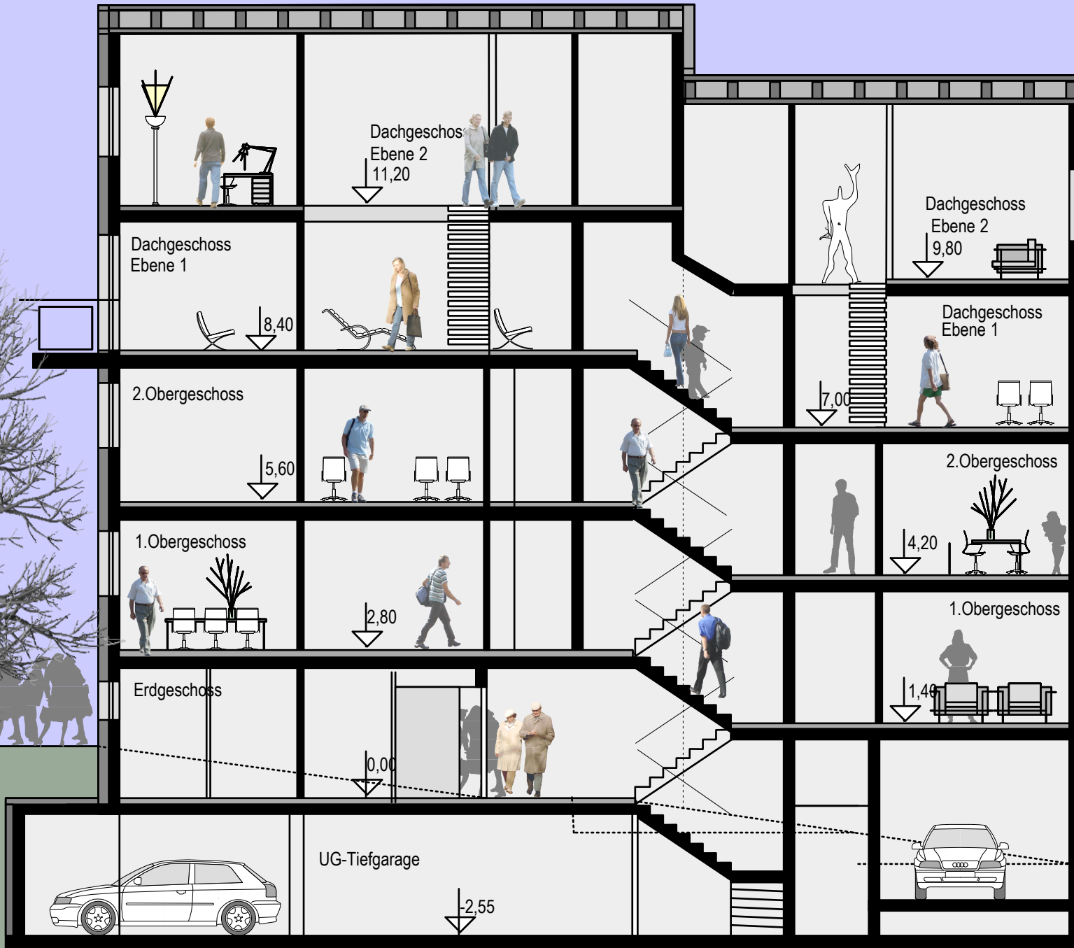
Längsschnitt M 1:100 Stuttgart-Sillenbuch "in der Werre 14 A-D"
