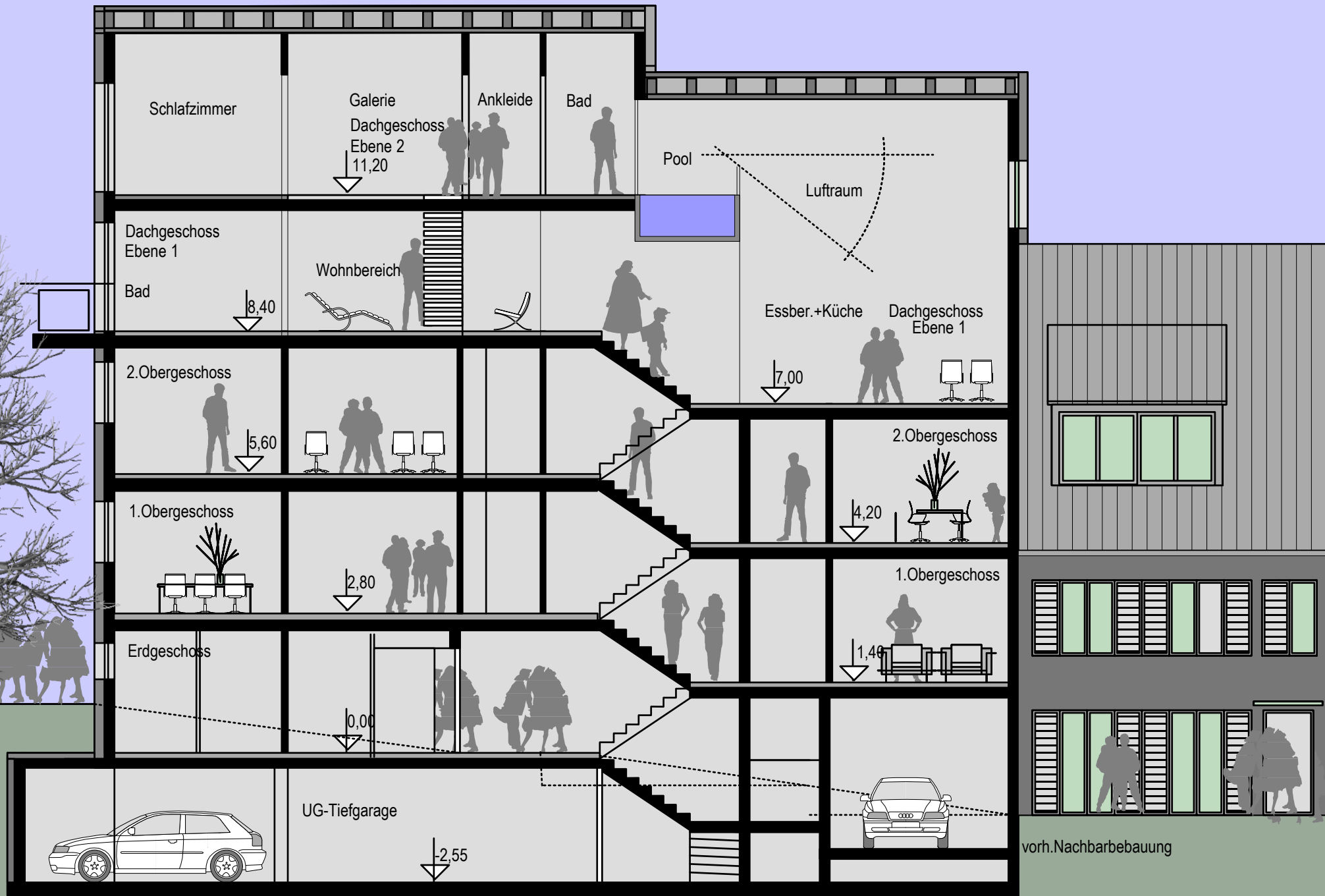
Längsschnitt mit Pool im Dachgeschoss M 1:100 Stuttgart-Sillenbuch "in der Werre 14 A-D"
